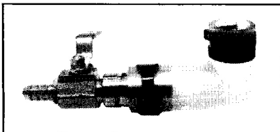
Anschlusset von 18 mm Pumpenanschluss zu 9 mm Kugelhahn und Luftschauchanschluss von 9 mm (art.nr. SC214)
