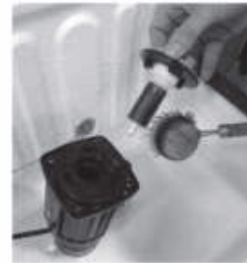
4. Laufrad vom Pumpengehäuse entfernen und mit Wasser und Bürste reinigen
